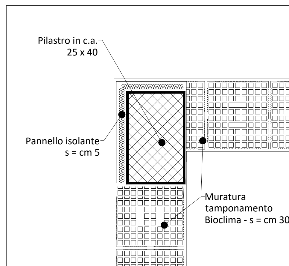
Particolare pilastro d'angolo
