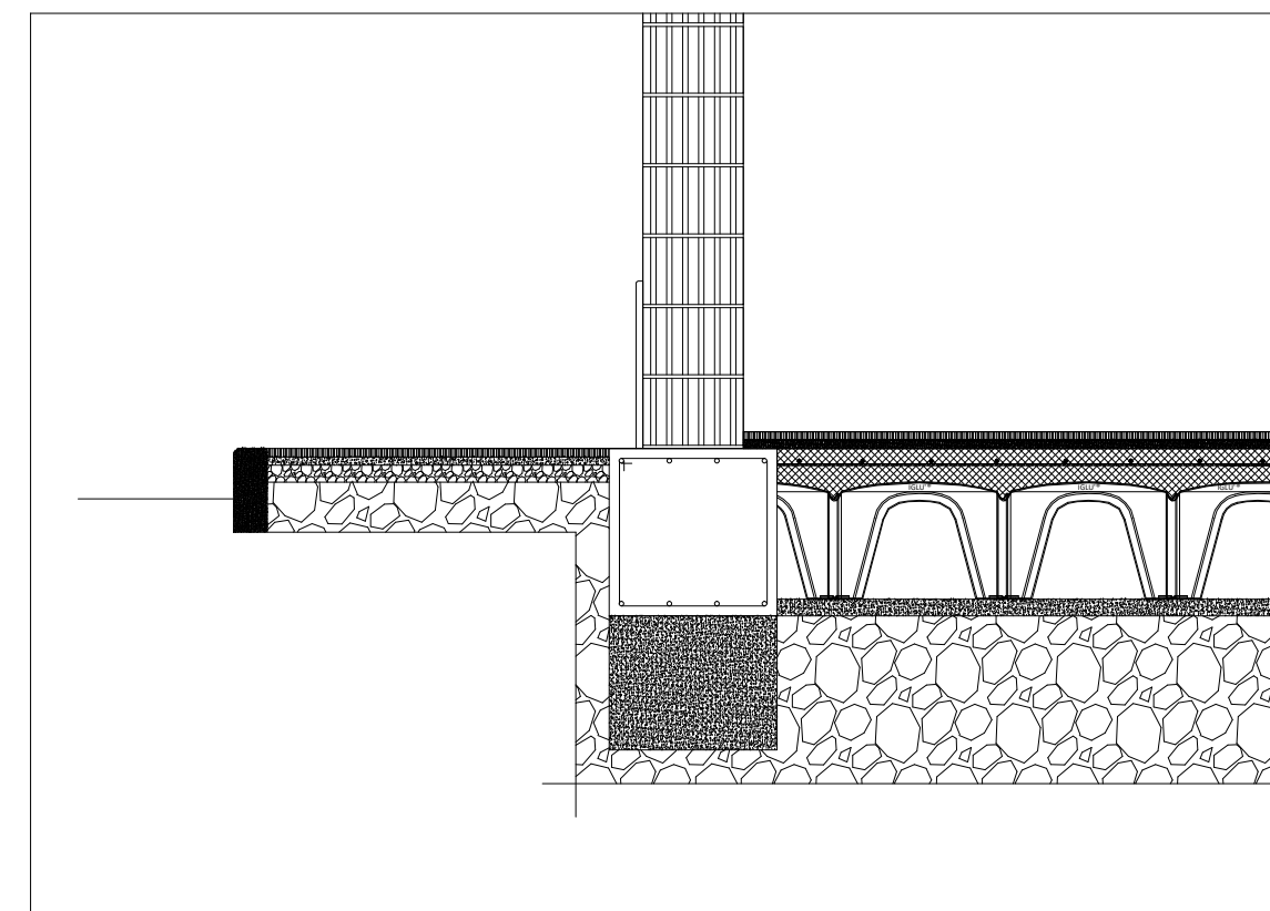
Particolare nodo muratura - pavimento
