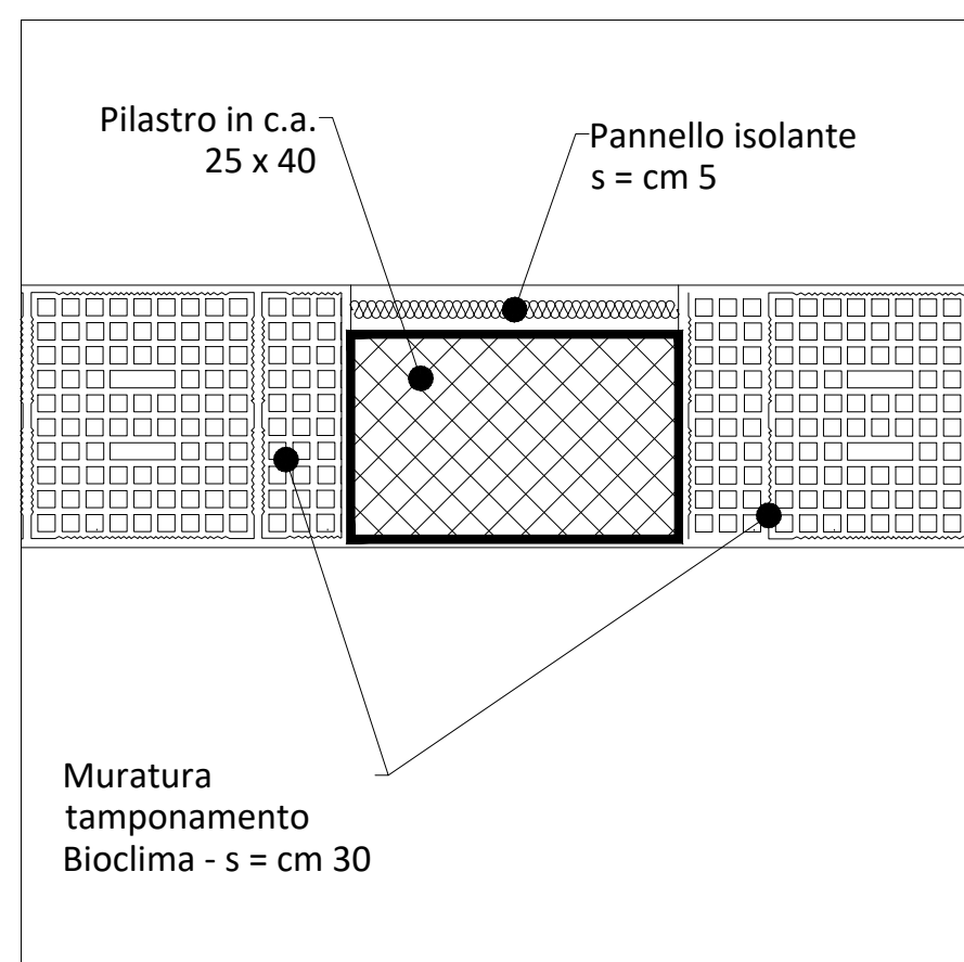
Particolare pilastro intermedio
